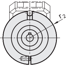
Ausführung für Lineareinheit Durchmesser 60"
