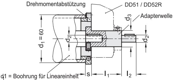
Ausführung für Lineareinheit Durchmesser 60"
